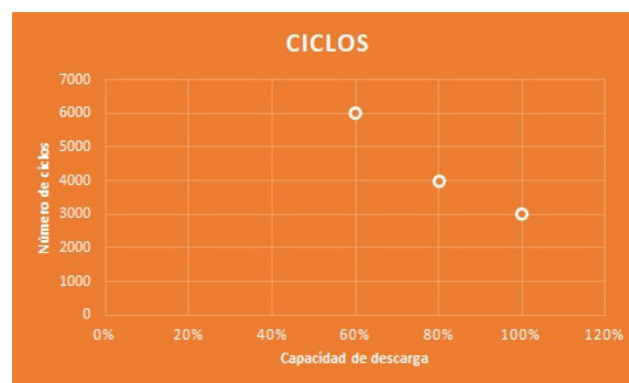
Curva de ciclo de vida vs descarga (1C)
